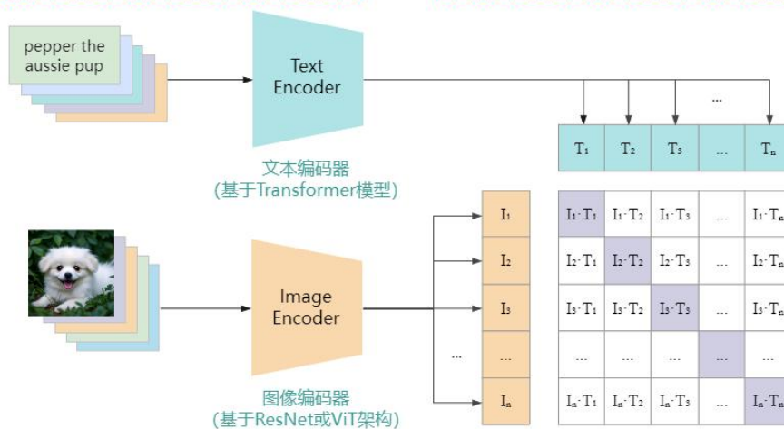
CLIP 模型结构图 (预训练阶段的)
